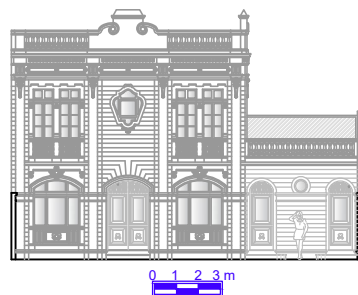
Elevation 01
